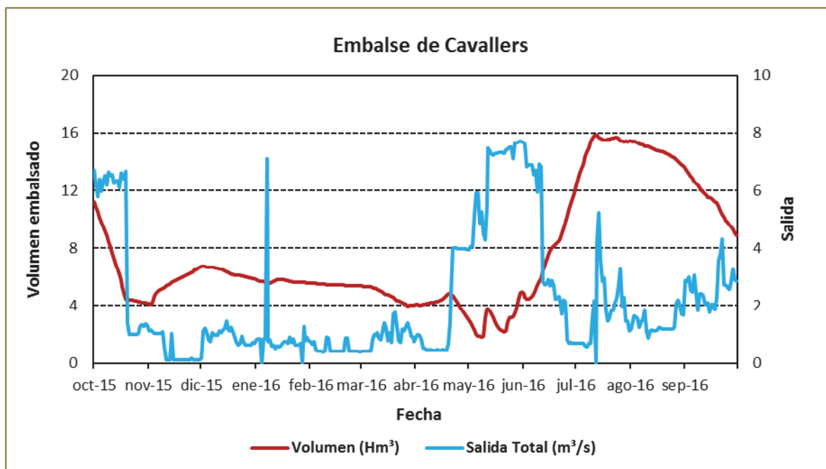
Figura 1. Volumen embalsado y salida durante el año hidrológico 2016-2015.
