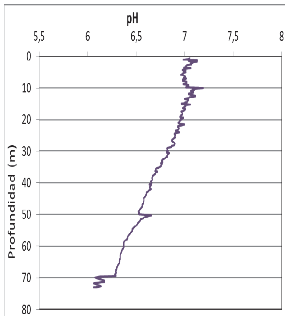
Figura 3. Perfiles verticales de la temperatura y pH.
