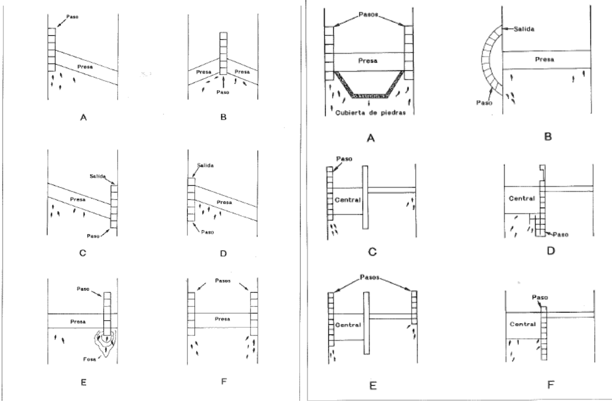
Figura 16. Disposición del paso en el obstáculo. A. Cubierta de piedras bajo el obstáculo para facilitar el acceso de los peces a los pasos. B. Situación del paso cuando existen problemas de espacio junto al obstáculo. C, D y E. Situación correcta del paso en un aprovechamiento hidroeléctrico. F. Situación incorrecta del paso en un aprovechamiento hidroeléctrico.
