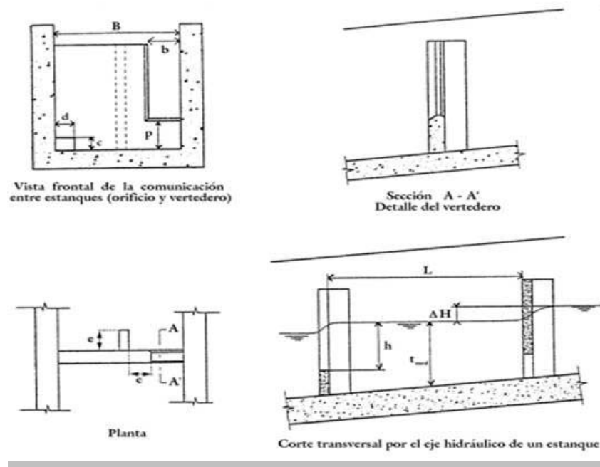
Fig. 12. Esquema de la artesa tipo.
