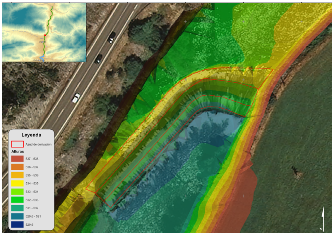
Fig. 8. Modelo digital del terreno en el entorno del azud
