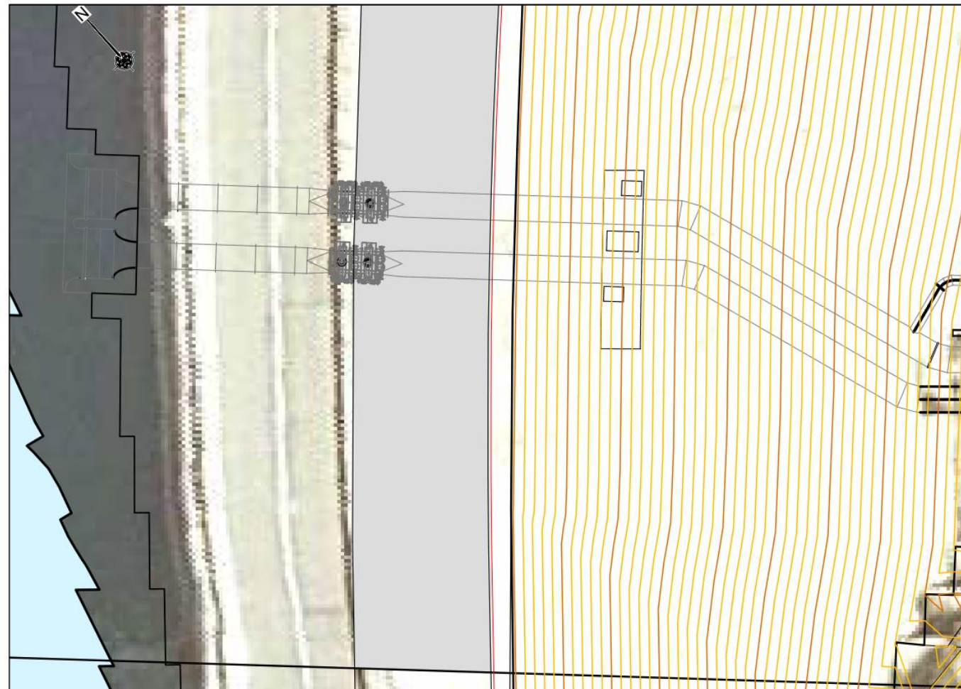
PLANTA DE TOMA ESCALA 1 : 250
